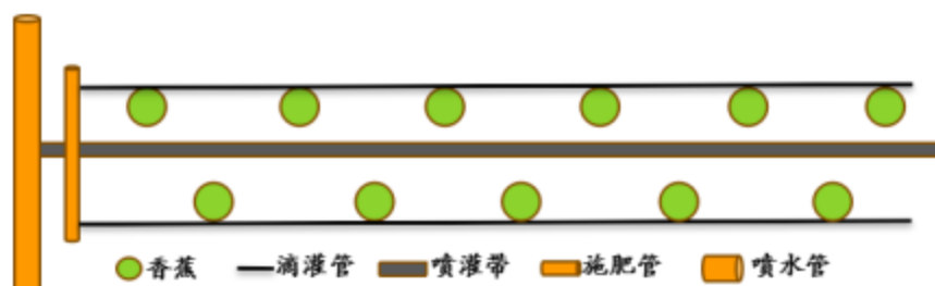
图 1 “一带双管”水肥一体化系统布置图
